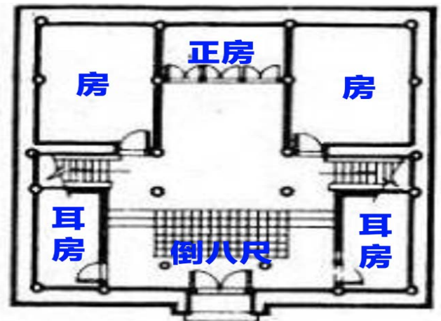
图一 一颗印中“三间两耳倒八尺”平面布局图
