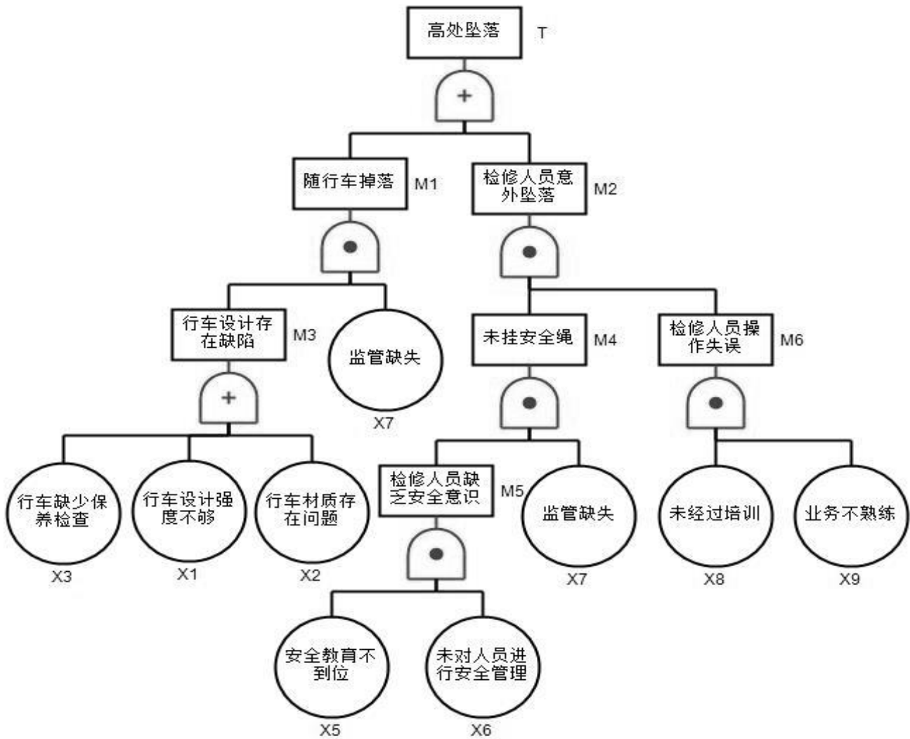
图4 高处坠落事故树分析图
