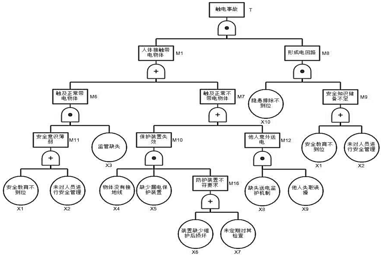
图 3 触电事故树分析图
