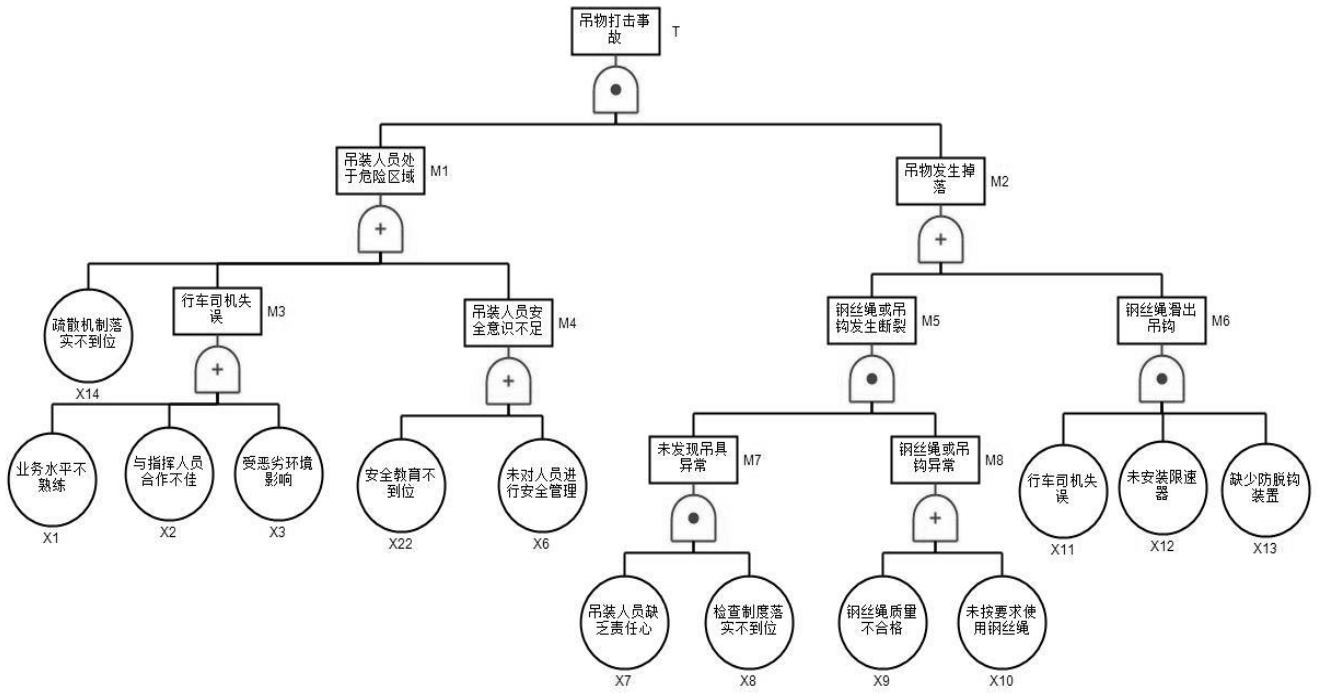
图 2 吊物打击事故树分析图
